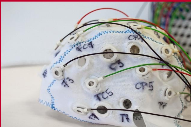
Elektroden-Kappe
