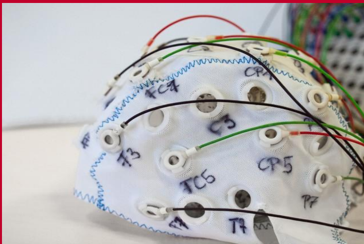
Elektroden-Kappe
